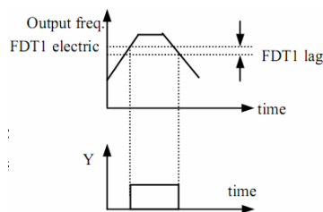
Рис.6-33 выявление уровня частоты
