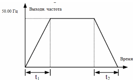
Рис. 6-3 Время ускорения/замедления
