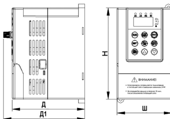
Рис.2-4 Общий вид
