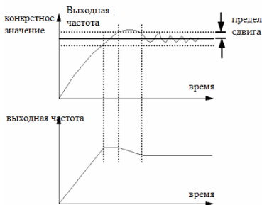
Рис. 6-17 предел сдвига
