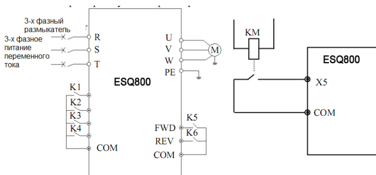
Рис. 6-25 работа на многоступенчатой скорости
