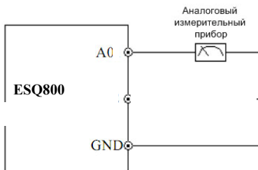
Рис. 3-10 Подключение проводов клеммной коробки аналогового вывода
