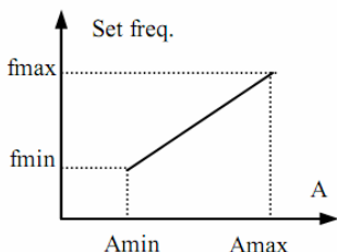
(1) положительная характеристика
