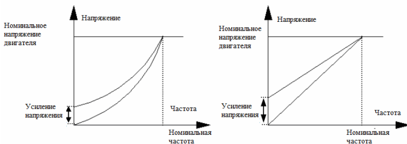
(а) график усиления вращающего момента, кривая замедления вращающего момента (b) график усиления вращающего момента, кривая постоянного вращающего момента
