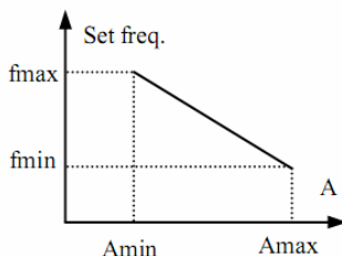
(2) отрицательная характеристика
