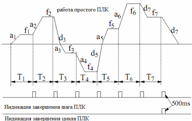
Рис. 6-19 работа простого ПЛК
