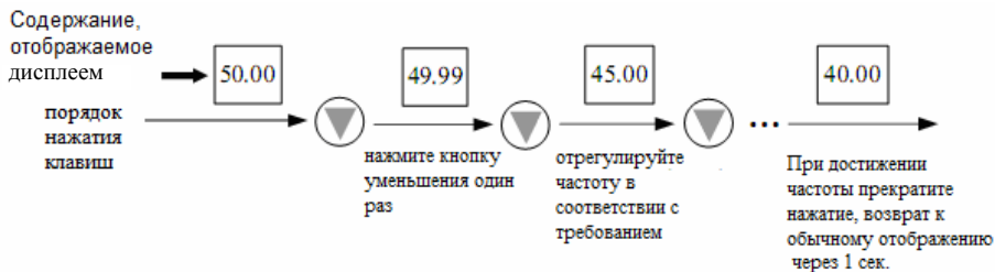
Рис. 4-8 Пример регулировки установленной частоты
