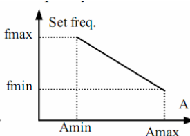
(2) отрицательная характеристика
