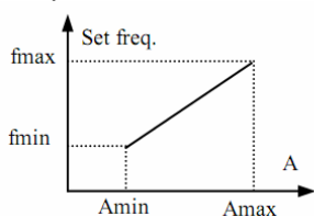
(1) положительная характеристика
