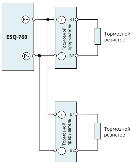
Рисунок 2-17. Параллельное подключение тормозных прерывателей
