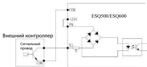
Рис.3-14 Режим подключения со встроенным источником питания на 24В 2. Для использования в преобразователь встроенного источника питания +24V и режима подключения внешнего контроллера типа PNP-сток.
