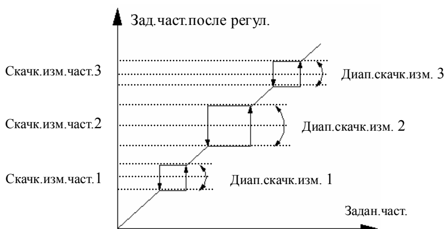
Рис.6-14 скачкообразное изменение частоты и диапазоны
