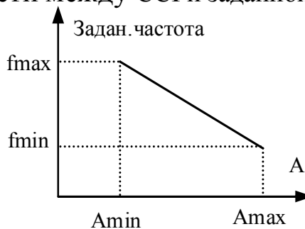
(2) отриц.харак-ка
