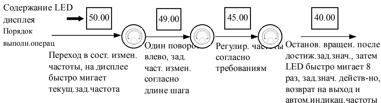
Рис. 4-8 пример регулировки заданной частоты
