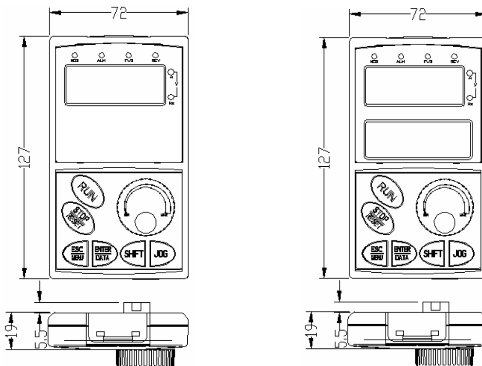
(a) Дистанционная панель KB3
