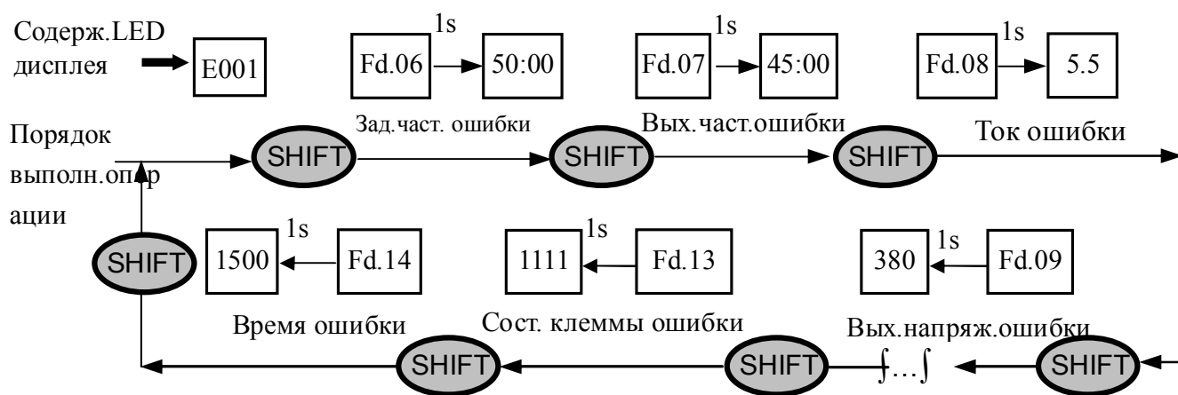
Рис.4-11 пример операции поиска состояния ошибки
