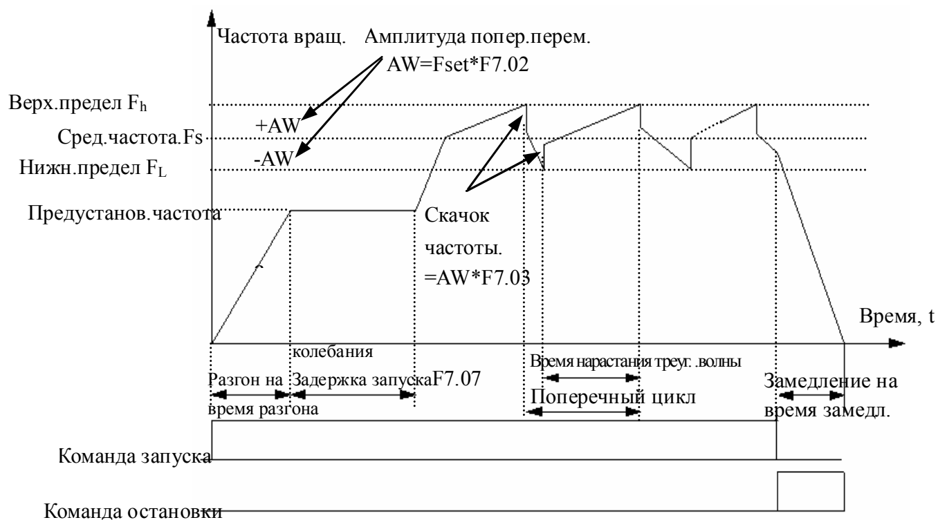
Рис. 6-41 Поперечное перемещение
