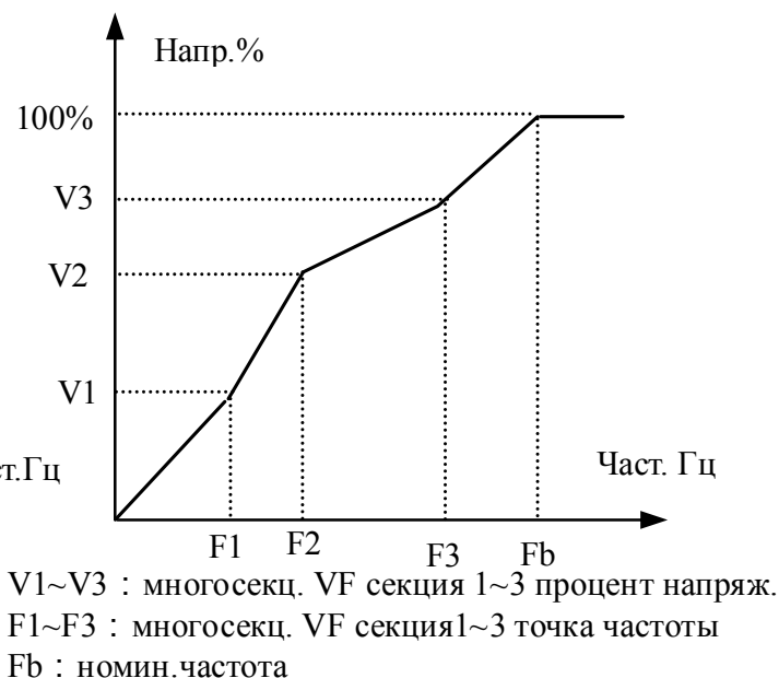
Рис.6-6 пользовательская V/F кривая
