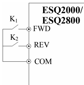
Рис.6-29 2-проводной режим 1
