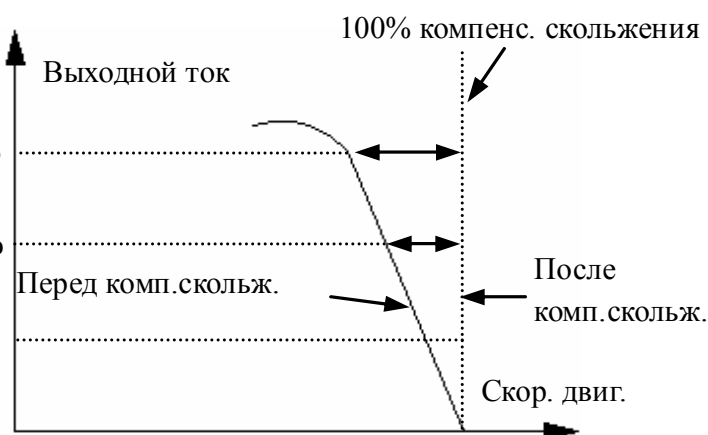
Рис.6-12 компенсация частоты скольжения
