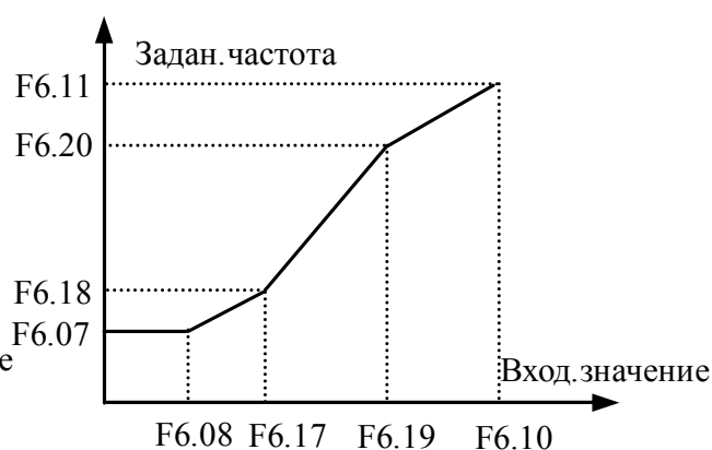
Рис. 6-40 Задан.частота 2, перегиб активен
