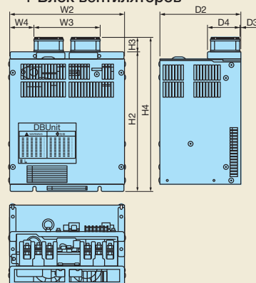
■ Тормозной модуль + Блок вентиляторов
