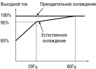
[Характеристика допустимого тока перегрузки]
