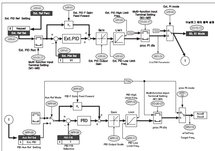
[Блок-схема двойного ПИД управления для случая ②]
