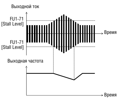
[Токоограничение при длительной работе]
