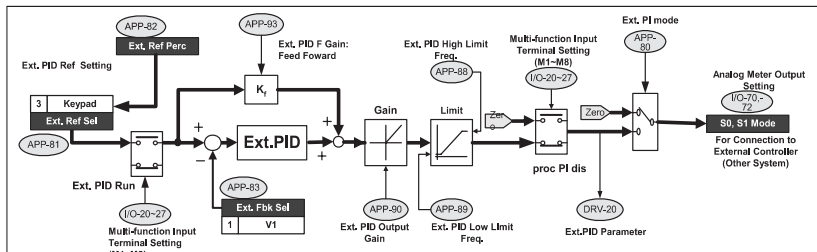
[Блок-схема двойного ПИД управления для случая ①]
