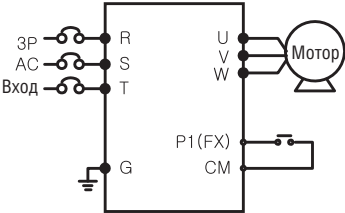
Схема подключения
