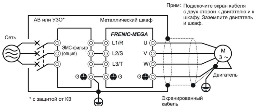
Рис. 9.3 Установка преобразователя частоты с ЭМС-фильтром в металлический шкаф
