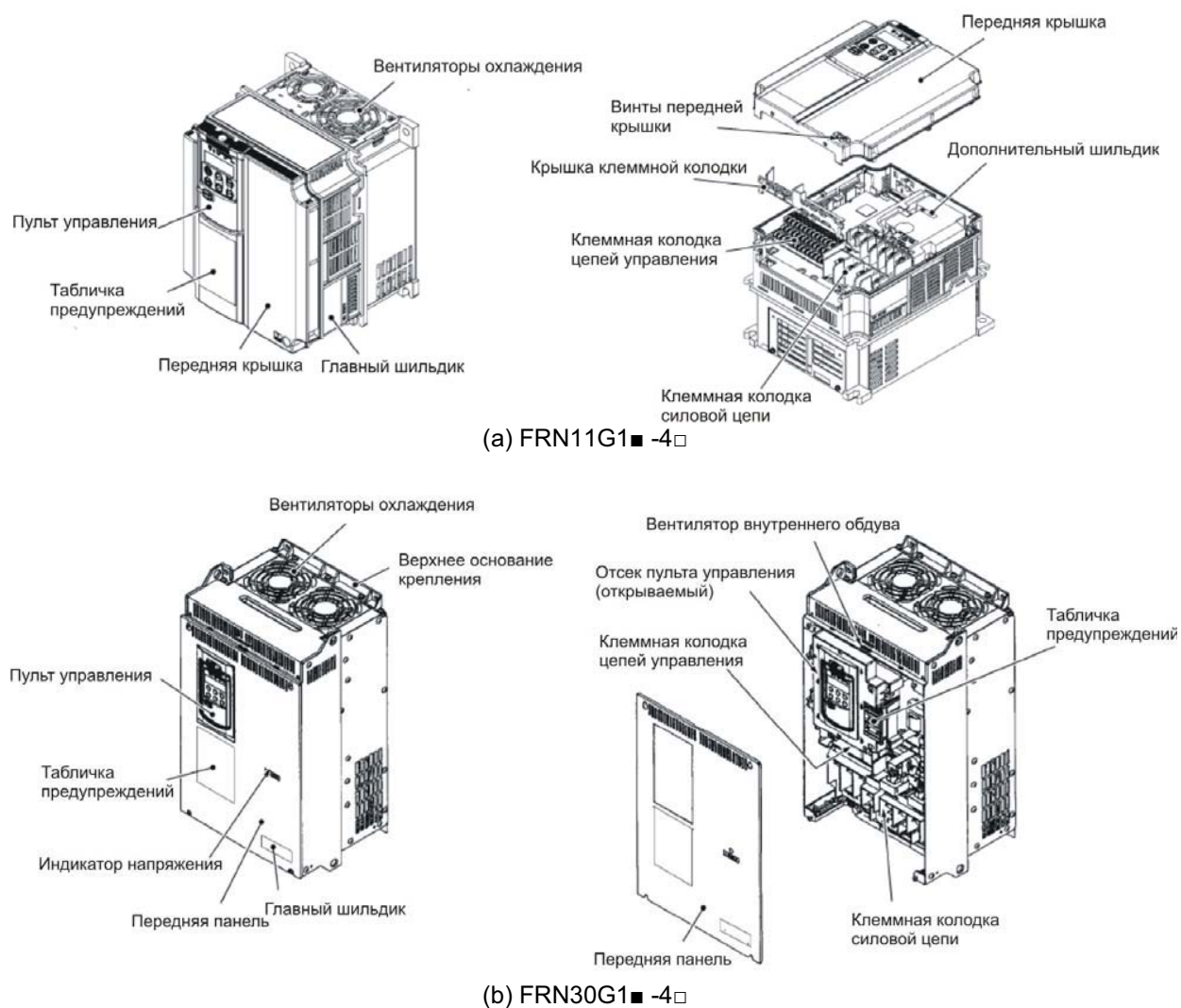
Рис. 1.2 Виды снаружи и внутри ПЧ
