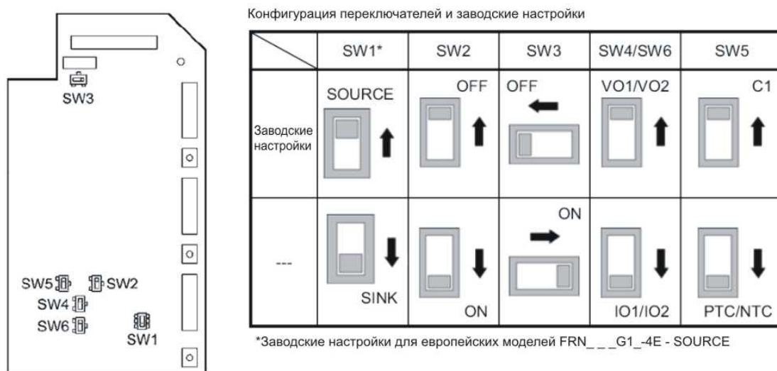
Рис. 2.19 Расположение микропереключателей на плате управления
