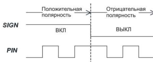
Полярность импульсного входа и направление вращения двигателя
