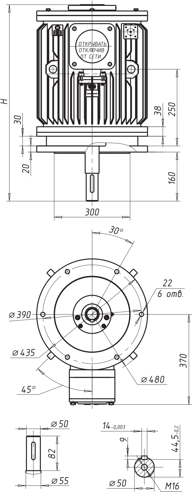
Рисунок 7. ВАСОУ-9 (-13, -15, -18,5) -12 (Монтажное исполнение IM 3011)
