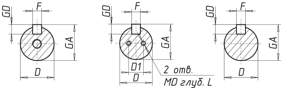
A-A исполнение 1
