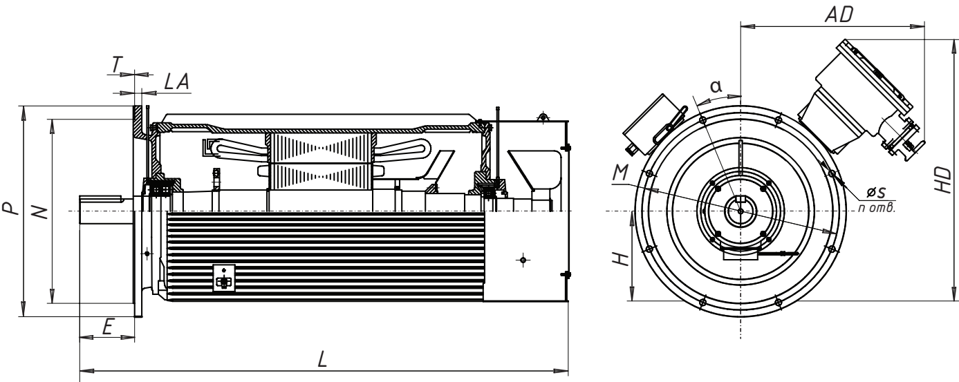
Монтажное исполнение IM 3001
