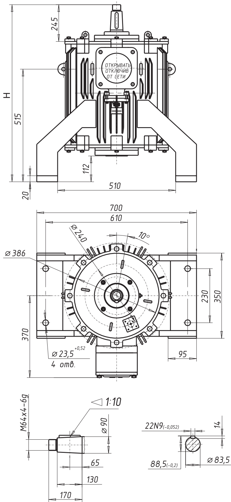
Рисунок 15. ВАСОУ-9 (-13, -15) -12 (Монтажное исполнение ИМ 9633) (сварные лапы)
