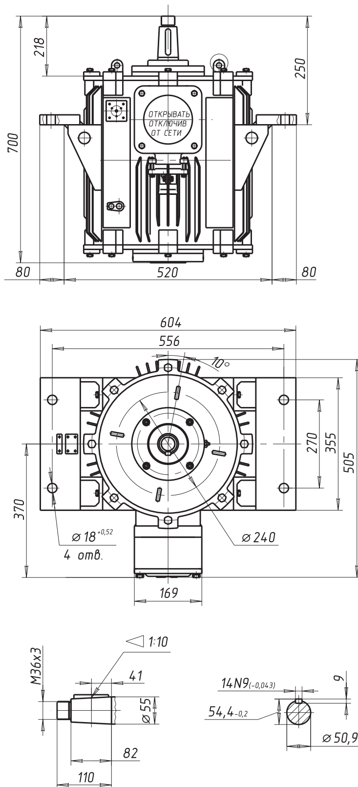
Рисунок 6. ВАСОУ-6,5-12 (Монтажное исполнение IM 9633) Масса - 185 кг
