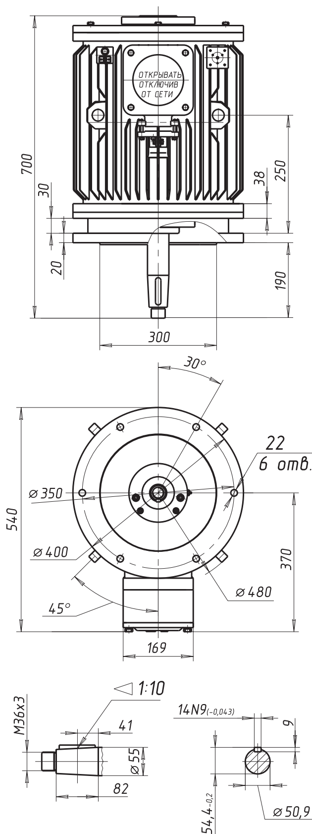
Рисунок 5. ВАСОУ-6,5-12 (Монтажное исполнение IM 3013) Масса - 185 кг
