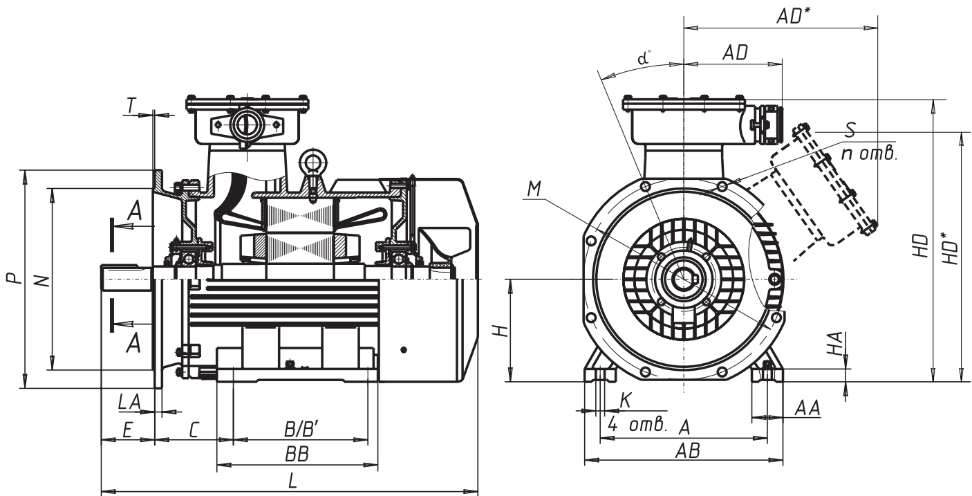
A-A исполнение 1
