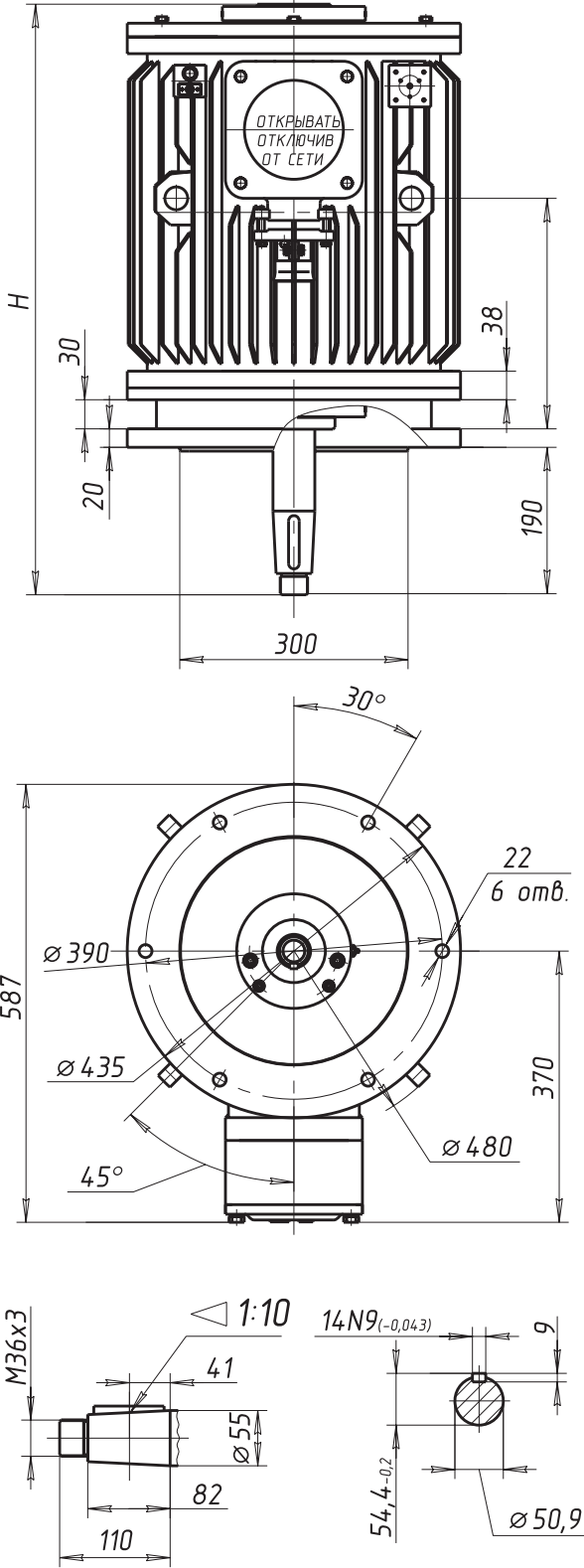
Рисунок 9. ВАСОУ-9 [-13, -15, -18,5] -12 (Монтажное исполнение IM 3013)
