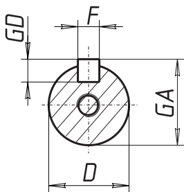
A-A исполнение 1
